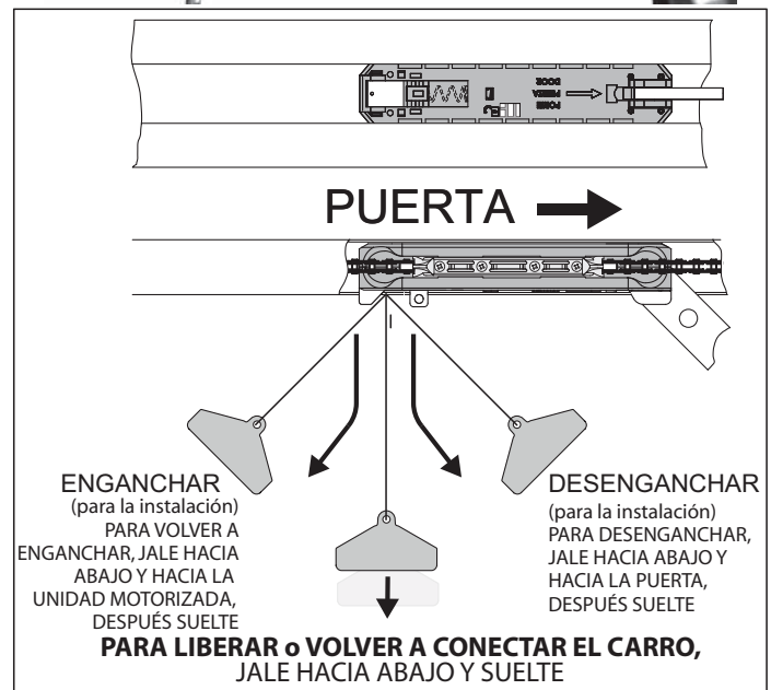
FIG. 6-4 Liberación del carro (vista transversal)
