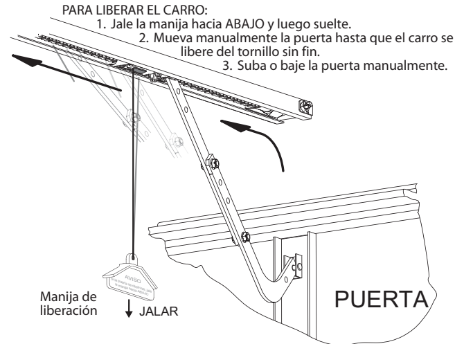
FIG. 6-3 Liberación del carro
