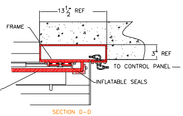
SECTION D-D
