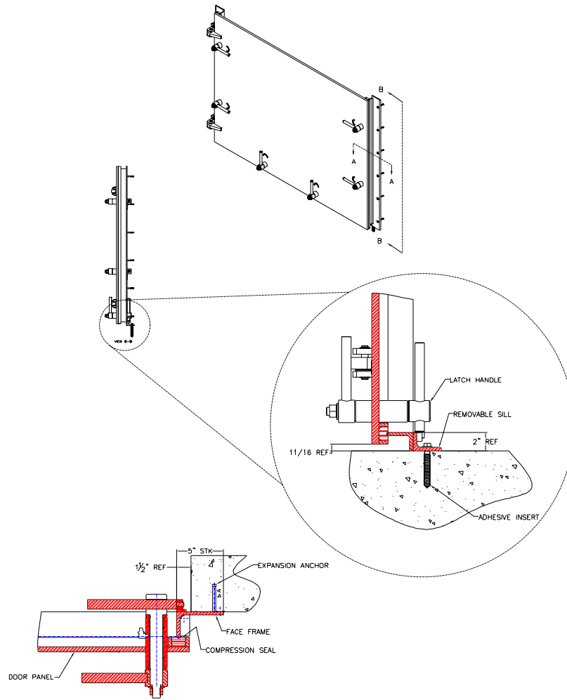
SECTION A-A
