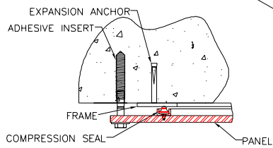
SECTION A-A TYP (4) SIDES
