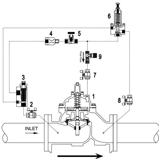
Schematic A-0423F
