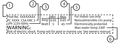
Fig. 6 Plaque signalétique
