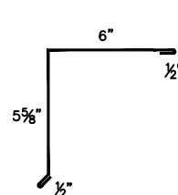
4b 2x4 MINI GABLE
