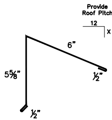
3b MINI TOP CAP
