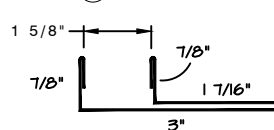
17) 24\" W-VALLEY
