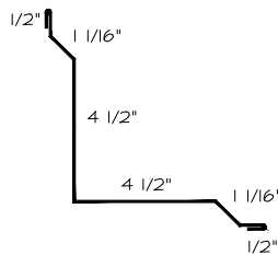
11) SNOW BREAK
