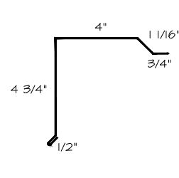
10) SIDEWALL
