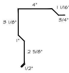
9) ENDWALL
