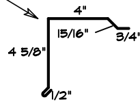
4b 2X4 MINI GABLE
