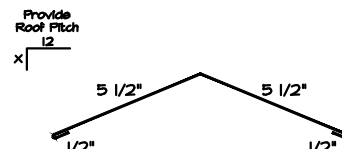
2) HIP RIDGE
