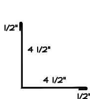
11) INSIDE CORNER
