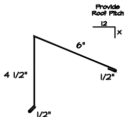
3b) 2x4 TOP CAP
