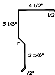
9) ENDWALL
