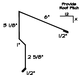
5b) 2x4 EAVE
