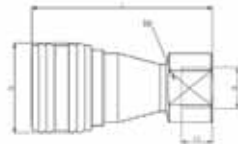
72KB POM Coupler
