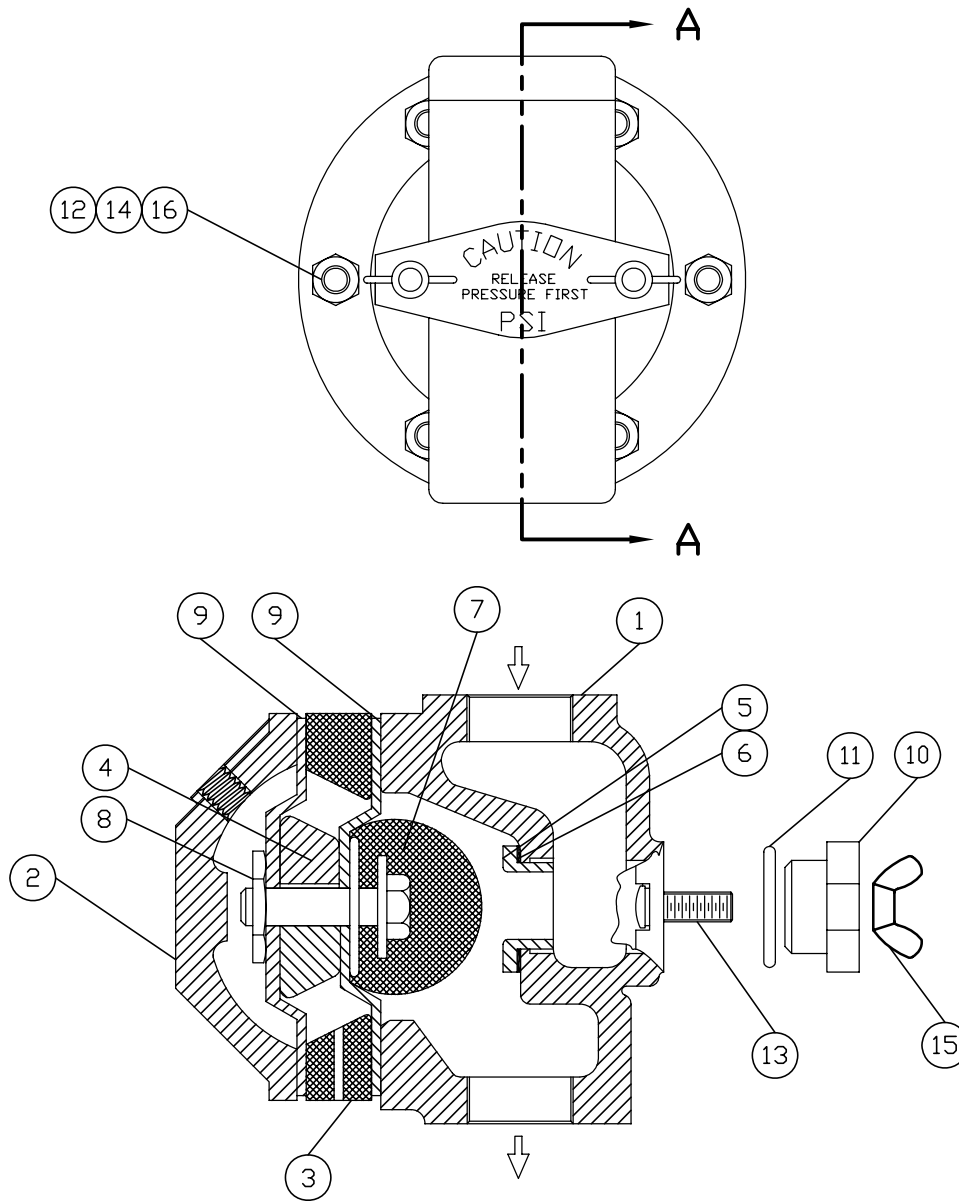
SECTION A-A
