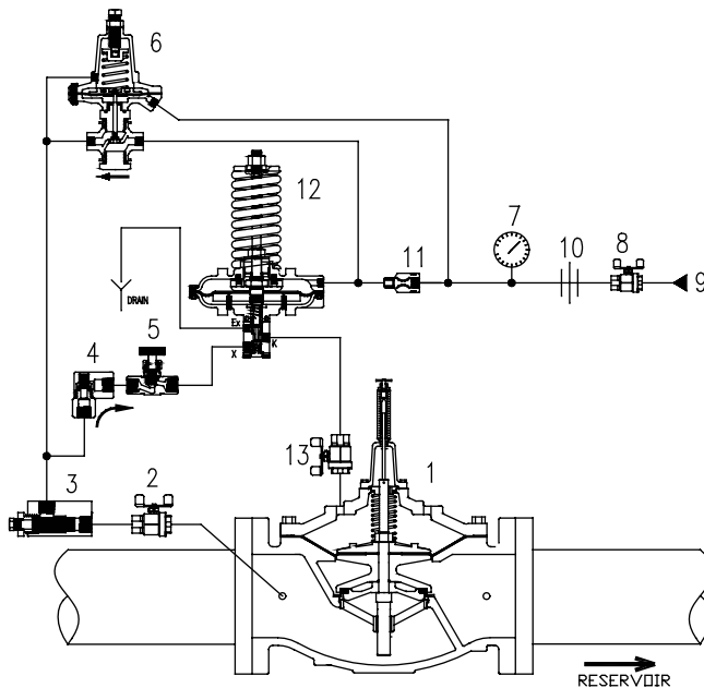
Schematic A-0414D
