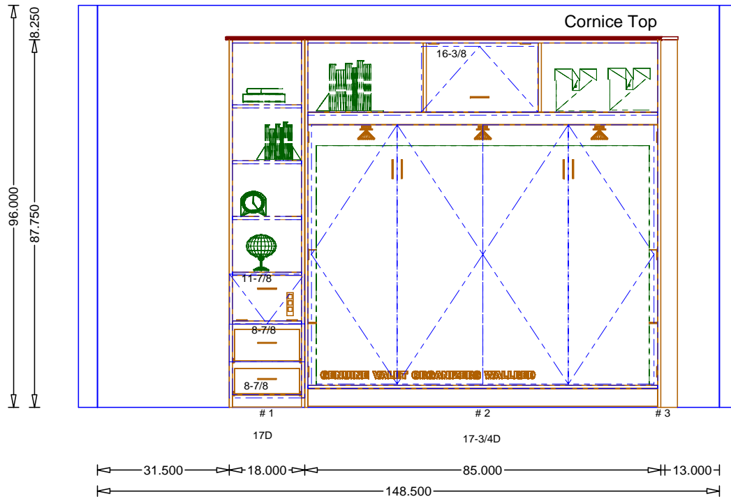
Elevation A
