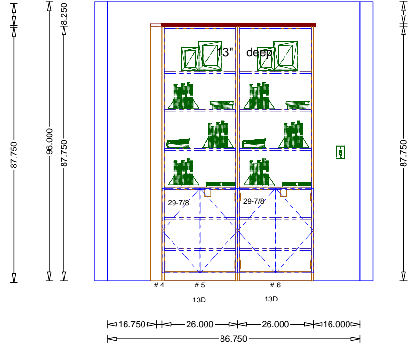
Elevation B
