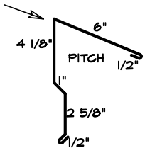
3a 2X6 TOP CAP
