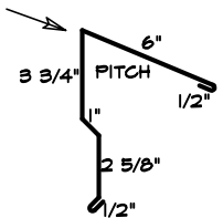
3a 2X6 TOP CAP
