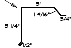
4b 2X4 MINI GABLE
