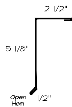
(9) ENDWALL
