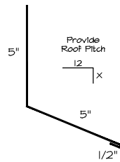
(9) ENDWALL
