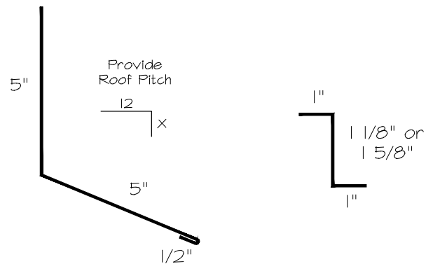
Endwall
