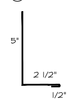
10a) SIDEWALL
