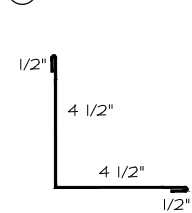
14) INSIDE CORNER
