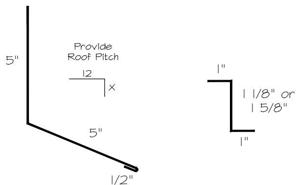
Endwall
