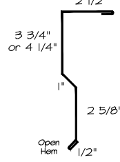
10a) SIDEWALL
