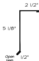
(9) ENDWALL
