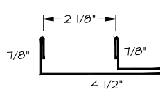
17) 24" W-VALLEY
