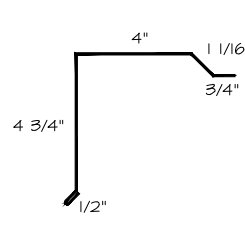
10) SIDEWALL
