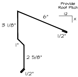
5b) 2x4 EAVE
