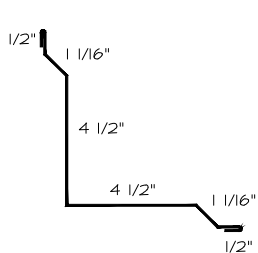
11) SNOW BREAK
