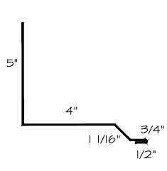
10) SIDEWALL
