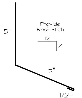
Endwall
