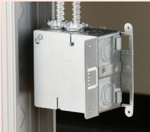
3 5/8" stud depth
