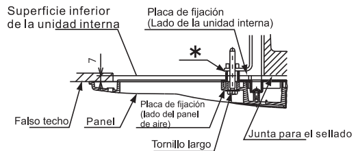
Imagen 2.3 Sección transversal del panel de aire
