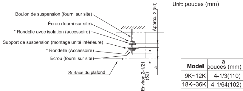
Fig.3.7 Écrous et rondelle de montage
