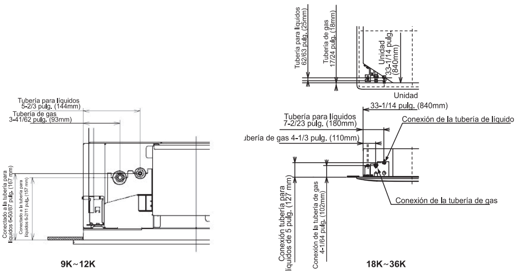
Fig. 4.1 Posición de la conexión de la tubería
