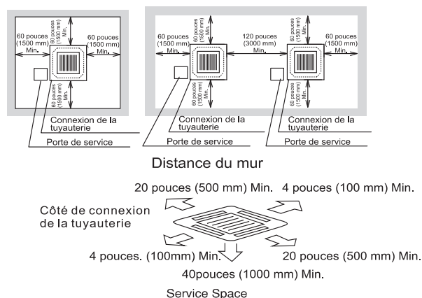
Fig. 3.1 Espacement autour de l'unité intérieure
