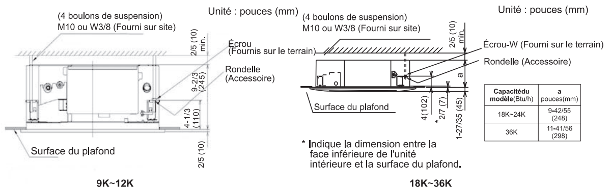
Fig 3.5 Position de montage
