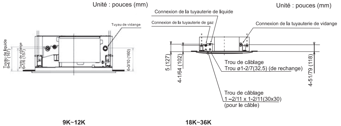
Fig. 3.6 Unité intérieure et panneau de régulation d'air
