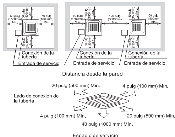
Fig. 3.1 Espacio alrededor de la unidad interior
