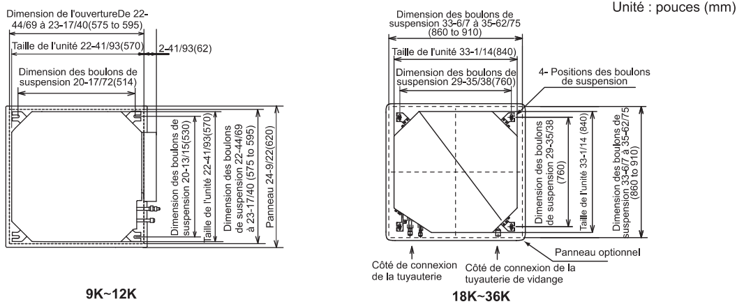
Fig.3.3 Ouverture des sous-plafonds et boulons de suspension
