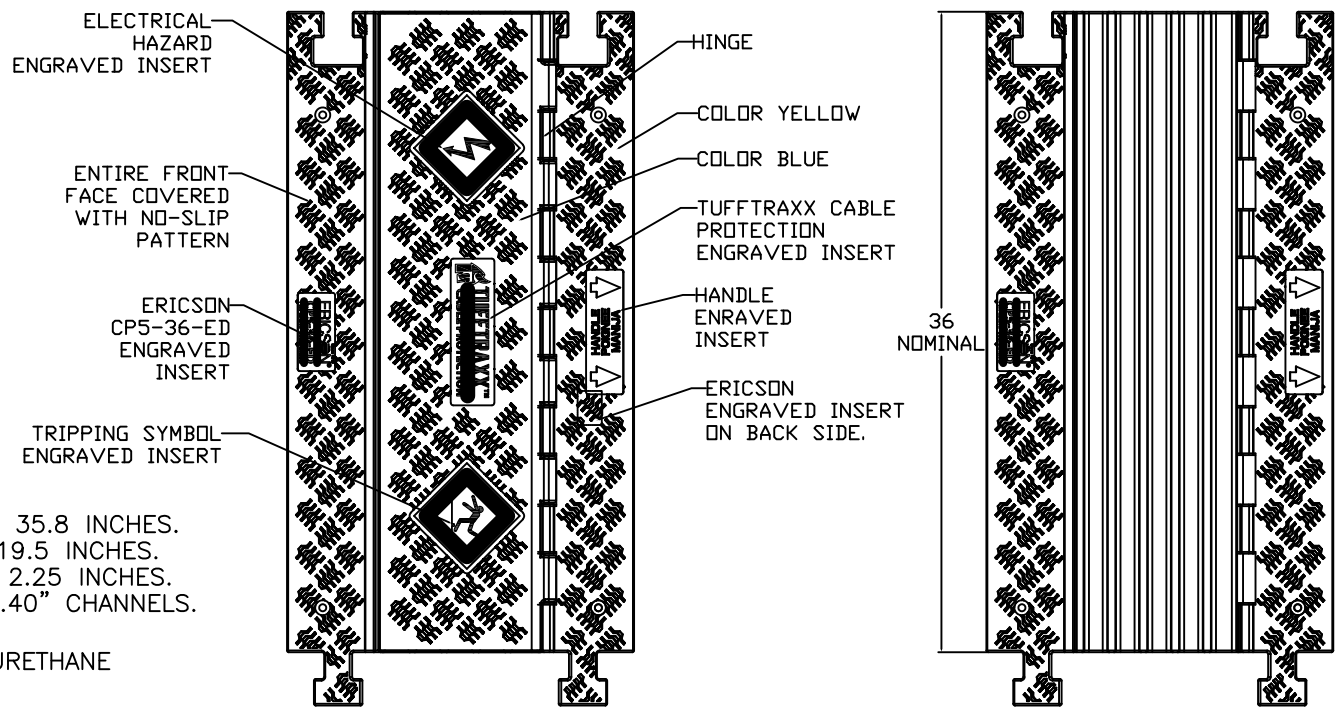
B2000561-1 LID AND B2000563-2 BASE
