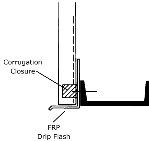
Jamb Detail
