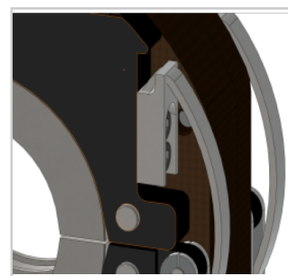
Verstellbares Federsystem berücksichtigt die Unrundheit der Rohre.
