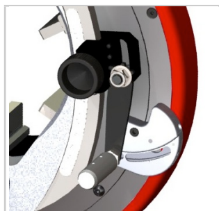
Sistema di guida profilo esterno: tiene conto dell'ovalizzazione dei tubi
