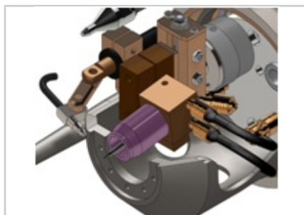
Testa inclinabile raffreddata ad acqua con filo inclinabile
