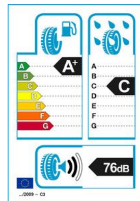
Reifenlabel Beispiel: Effizienzklasse A+, Nasshaftung C, Geräuschemission 2 Streifen, Geräuschemission in Dezibel 76dB, Fahrzeugklasse C3
