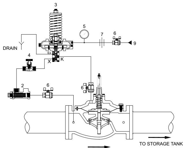
Schematic A-0413C
