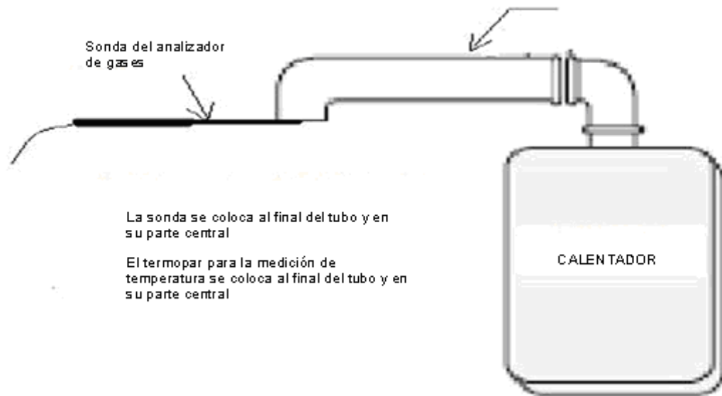
FIGURA 5 b)-Equipo para el análisis de CO en calentadores provistos de ducto (ilustrativa no limitativa)
