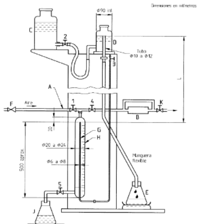
FIGURA A.1. Dispositivo para la verificación de la hermeticidad del circuito de gas (Método volumétrico) (Ver 7.9 y Apéndice A)
