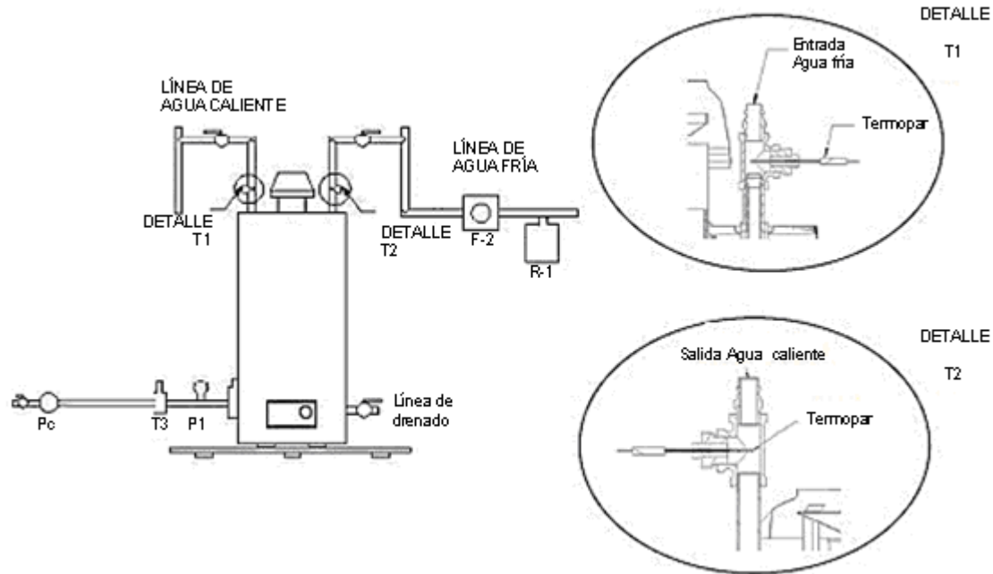
FIGURA 2 Calentador de rápida recuperación (ilustrativa no limitativa)
