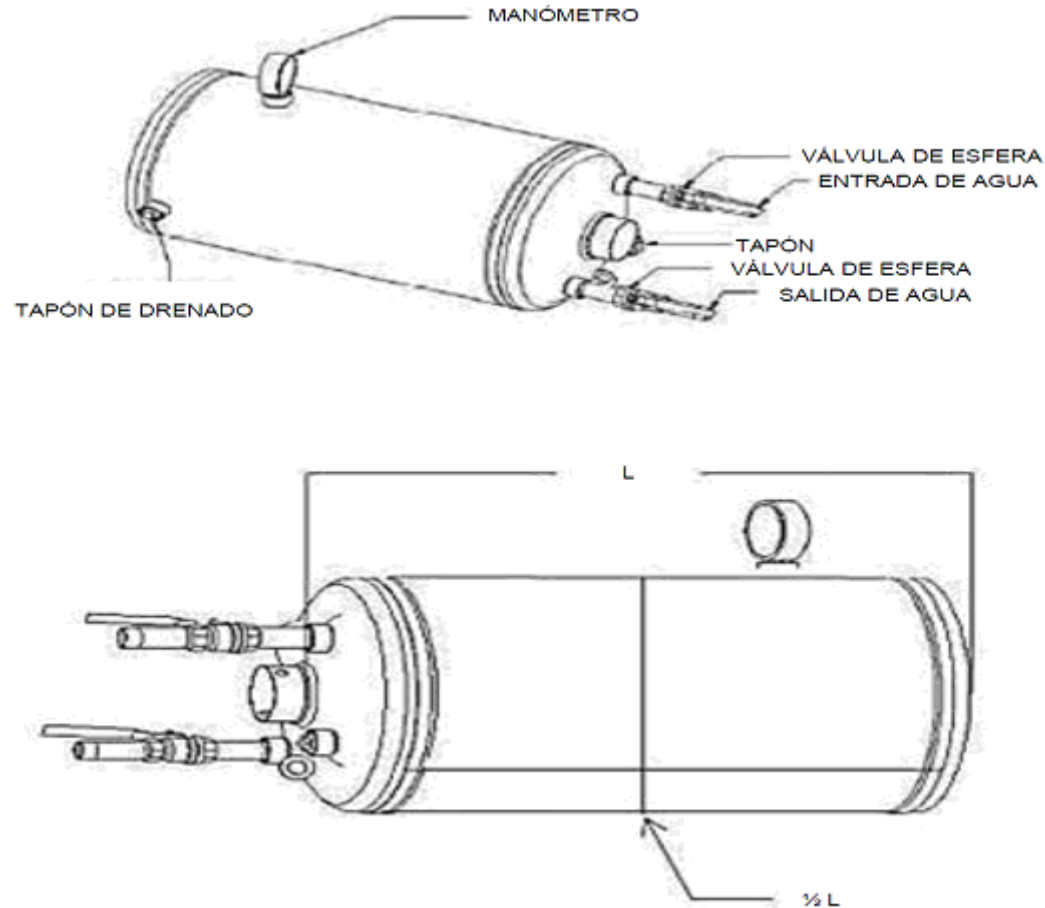
FIGURA 4-Exterior del calentador (ilustrativa no limitativa)
