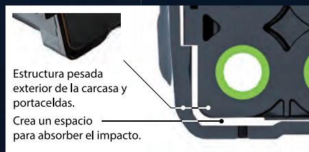
Estructura de absorción de impacto.
