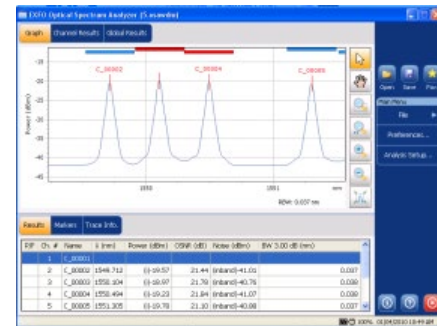
Ein OSA misst die Leistung gegen Wellenlänge Inclusive OSNR & \lambda
