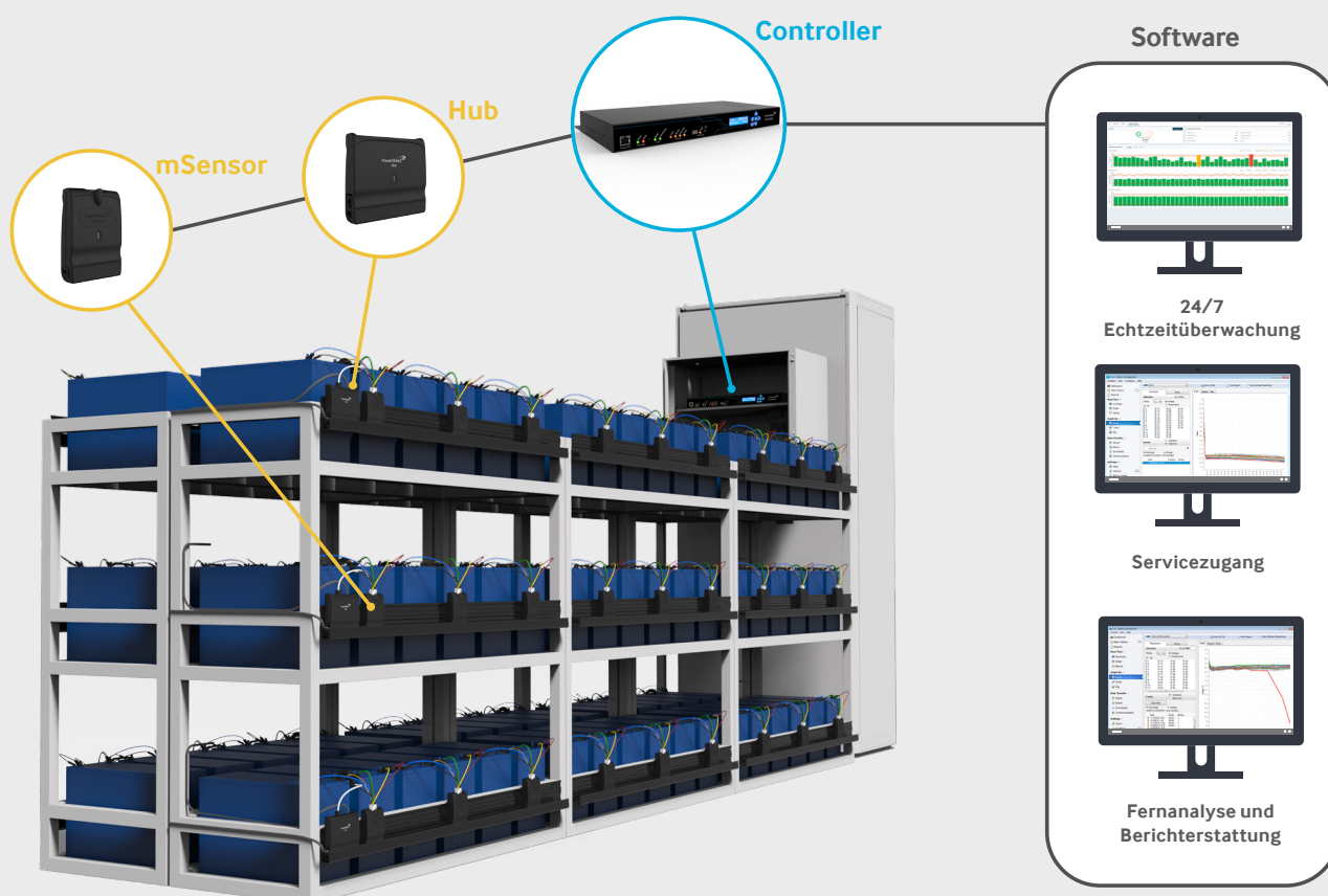
Abbildung 1. Typische Konfiguration des Batteriemangementystems PowerShield 8
