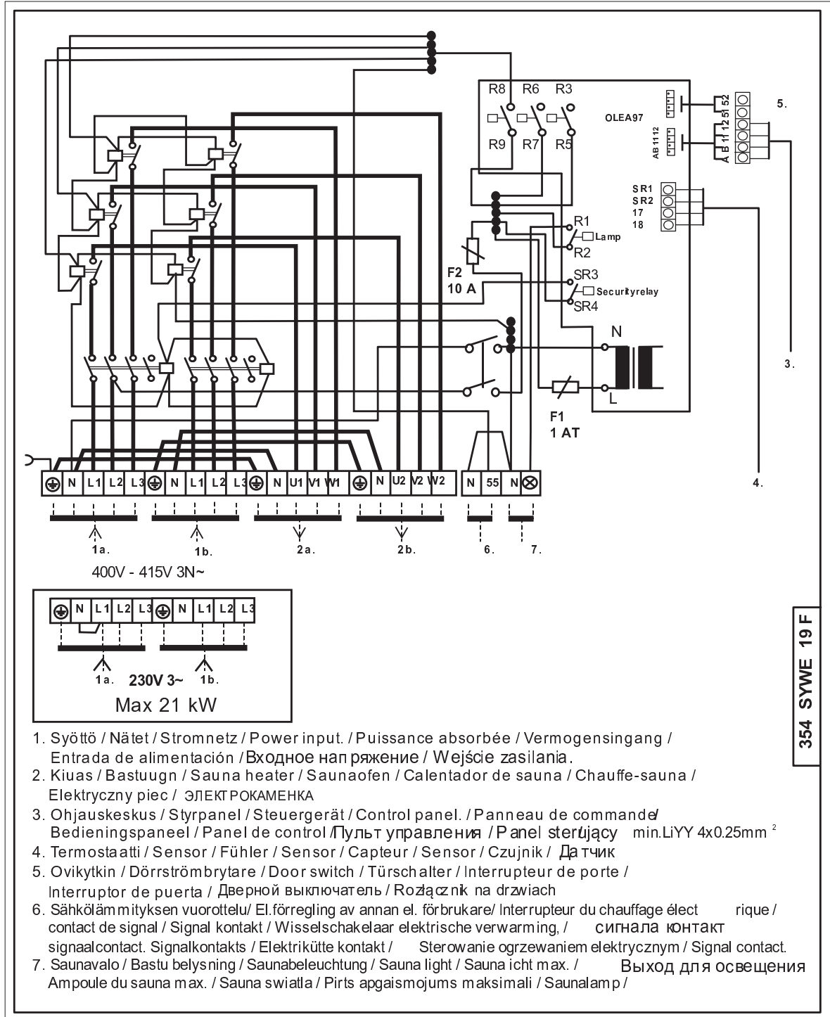
Bild. 5 Kopplingschema WE 14
