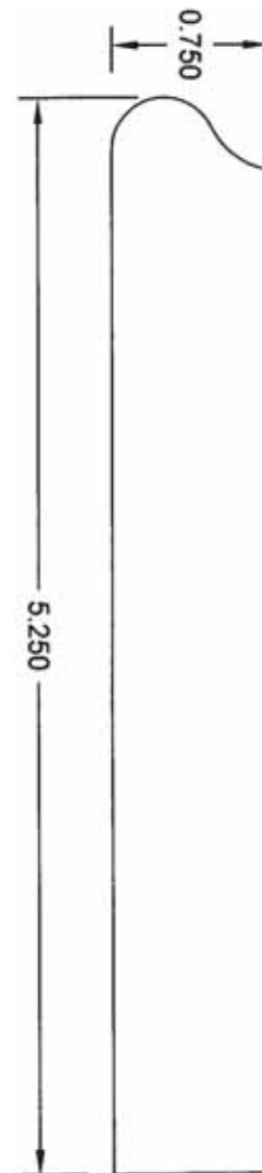
5 1/4" Stool BL68
