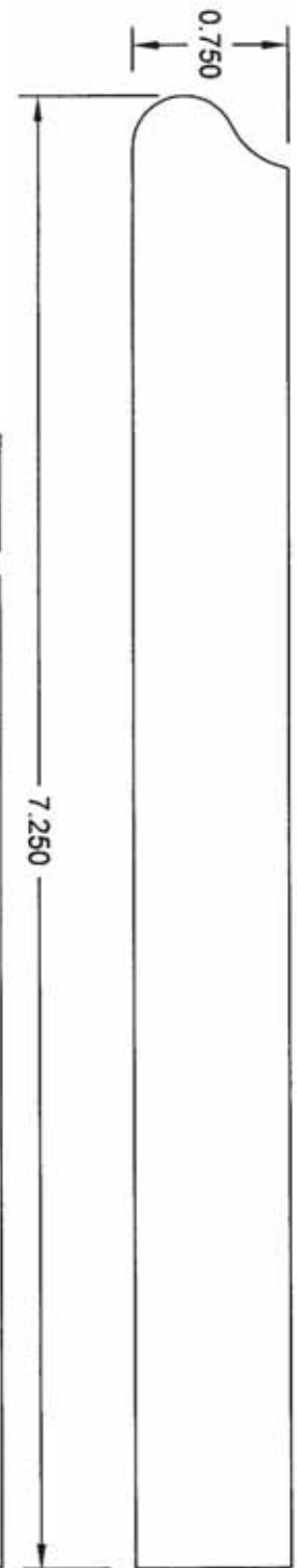
7 1/4" Stool BL69
