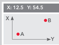
GEOCODING
