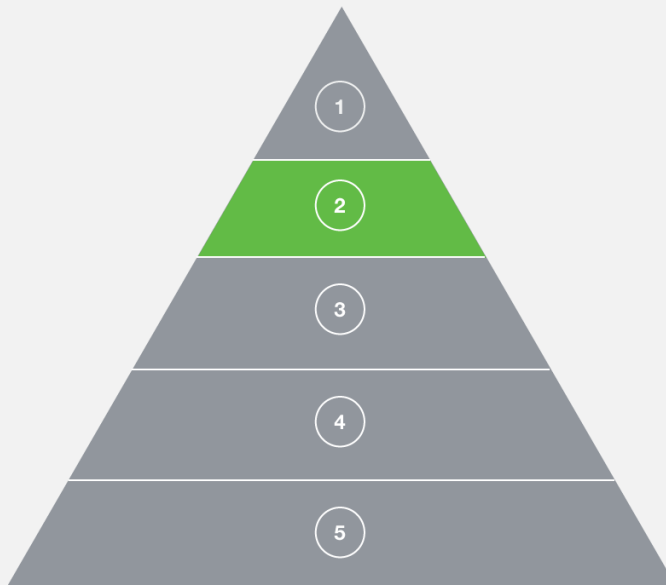
Message hierarchy
