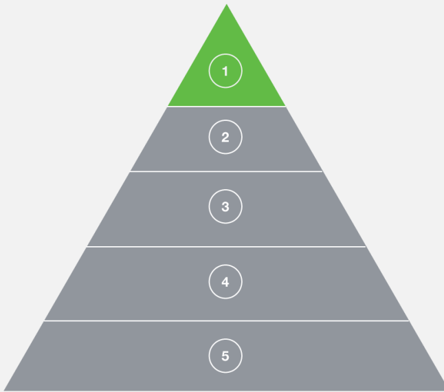
Message hierarchy
