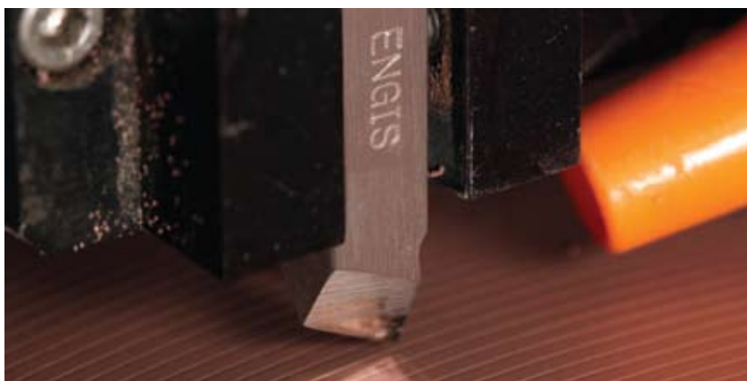
图 3 修面机构用金刚石刀具切除研磨盘最上层 (已磨损), 并将研磨盘修至数微米内的平面度, 简化了磨盘修复过程。
