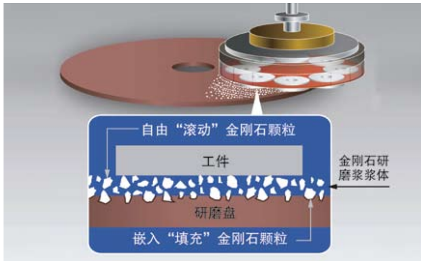
图 1 嵌入的和自由的金刚石颗粒混合作用于研磨过程
