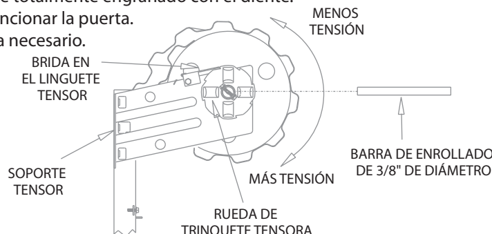
FIGURA 11 AJUSTE DE LA TENSIÓN DEL RESORTE
