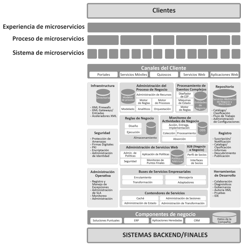
Figura 3: En un escenario de “microservices washing”, la arquitectura de microservicios real es de hecho más complicada de lo que se describe. Este diagrama es a menudo como realmente funciona.
