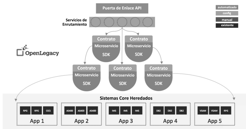
Figura 2. Algunos proveedores (como OpenLegacy) evitan capas de arquitectura para conectarse directamente con los sistemas monolíticos heredados existentes. Además, muchos procesos manuales están automatizados, simplificando y acelerando así el proceso.
