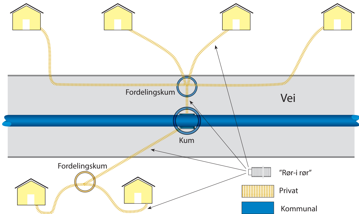
Ny løsning for private vannledninger
