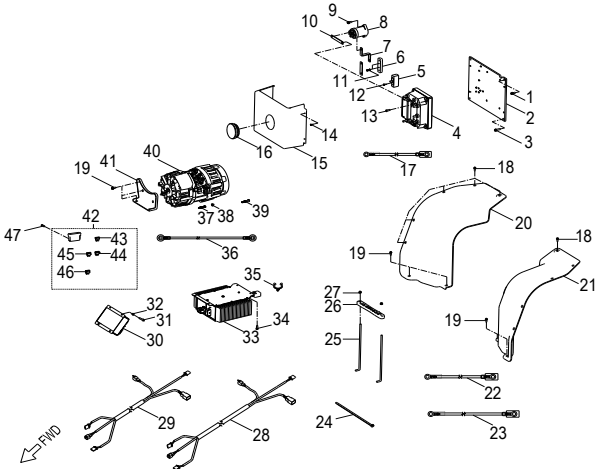
D-26:ELECTRIC MOTOR
