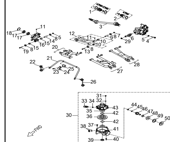
D-21:SWING ARM
