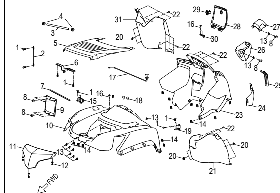
D-6:CAB
