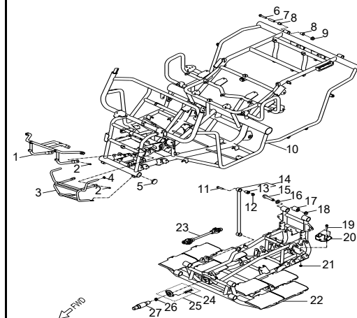
D-3:FRAME BODY
