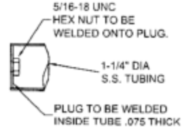
Detail of Stud End
