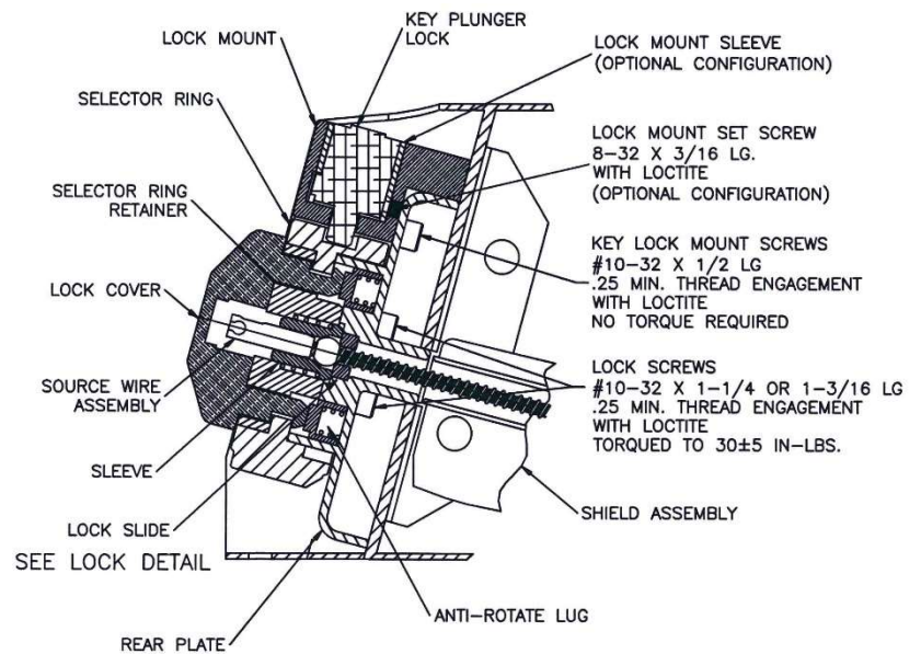
SECTION D-D
