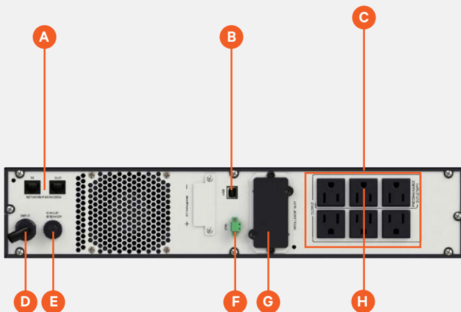
PSI5-1500RT120LI
